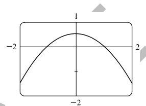
e = 1
